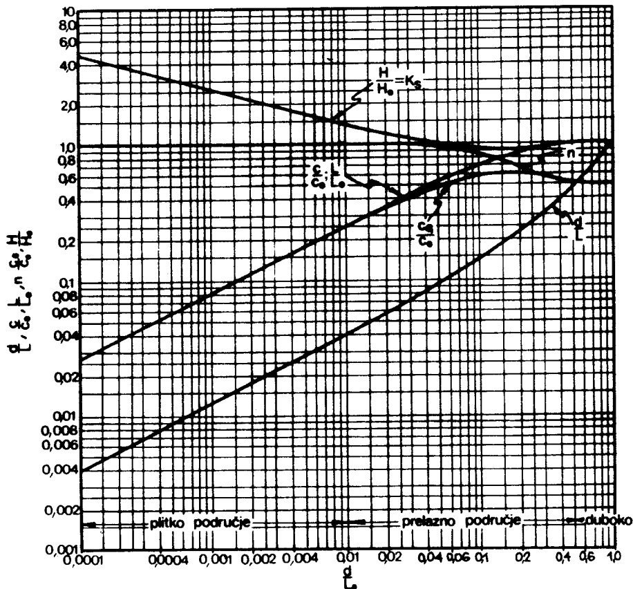
Sl. 1.2 - 5.2::3 Funkcije od d/L_0 prema linearnoj teoriji, Wiegel 1948. [3]
