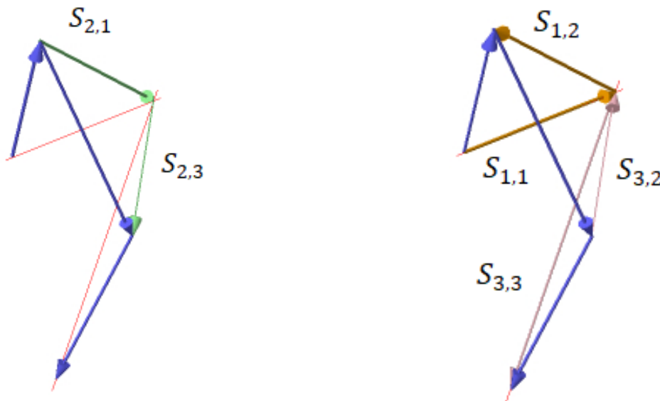
Slika 24.: Komponente sila \vec{S}_1 i \vec{S}_3
